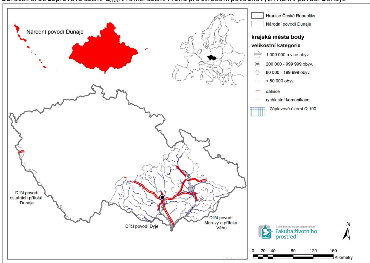
Obrázek č. 16 Záplavová území Q_{100} v rámci území Plánu pro zvládnání povodňových rizik v povodí Dunaje
