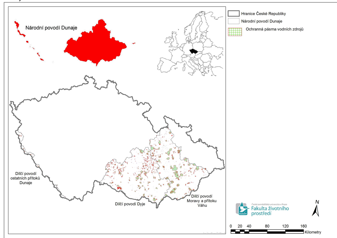
Obrázek č. 15 Ochranná pásma vodních zdrojů v rámci území Plánu pro zvládnání povodňových rizik v povodí Dunaje
