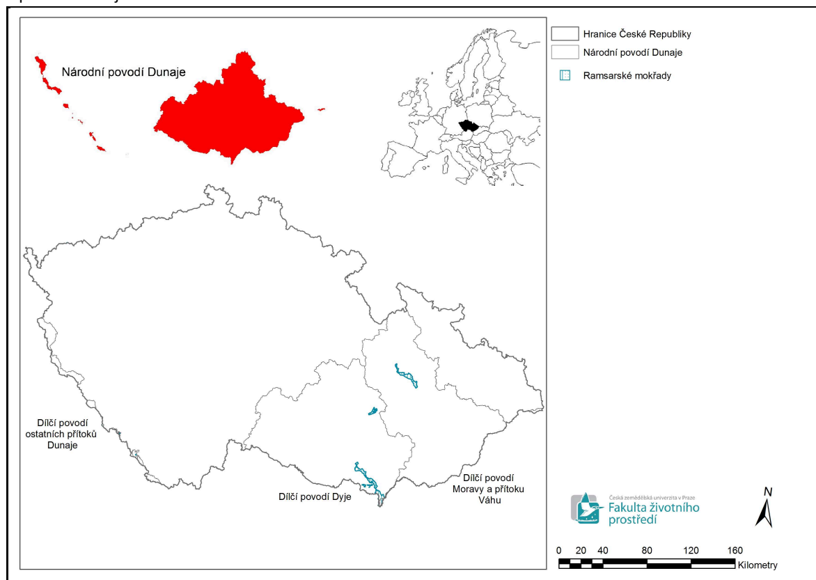
Obrázek č. 14 Území chráněné Ramsarskou konvencí v rámci území Plánu pro zvládnání povodňových rizik v povodí Dunaje
