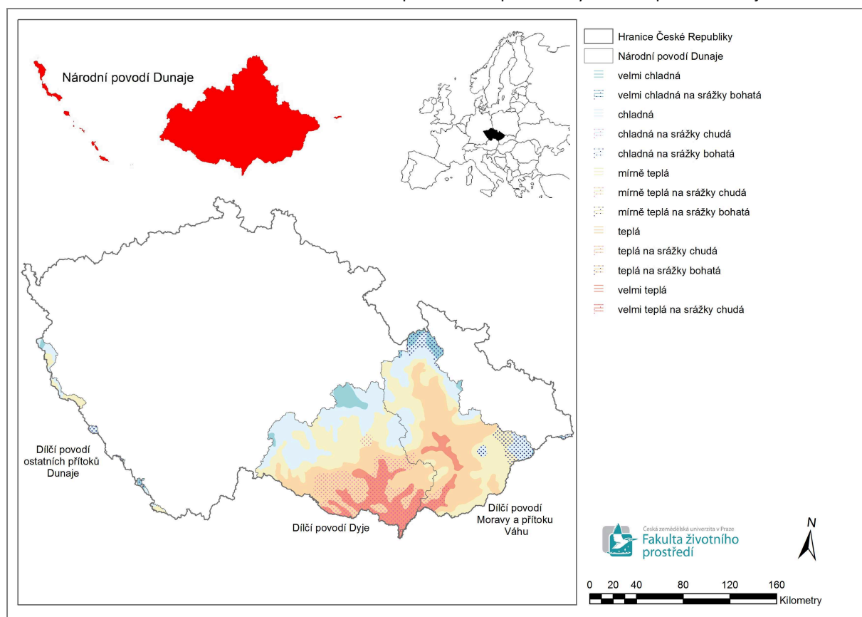
Obrázek č. 4 Klimatické oblasti v rámci území Plánu pro zvládnutí povodňových rizik v povodí Dunaje
