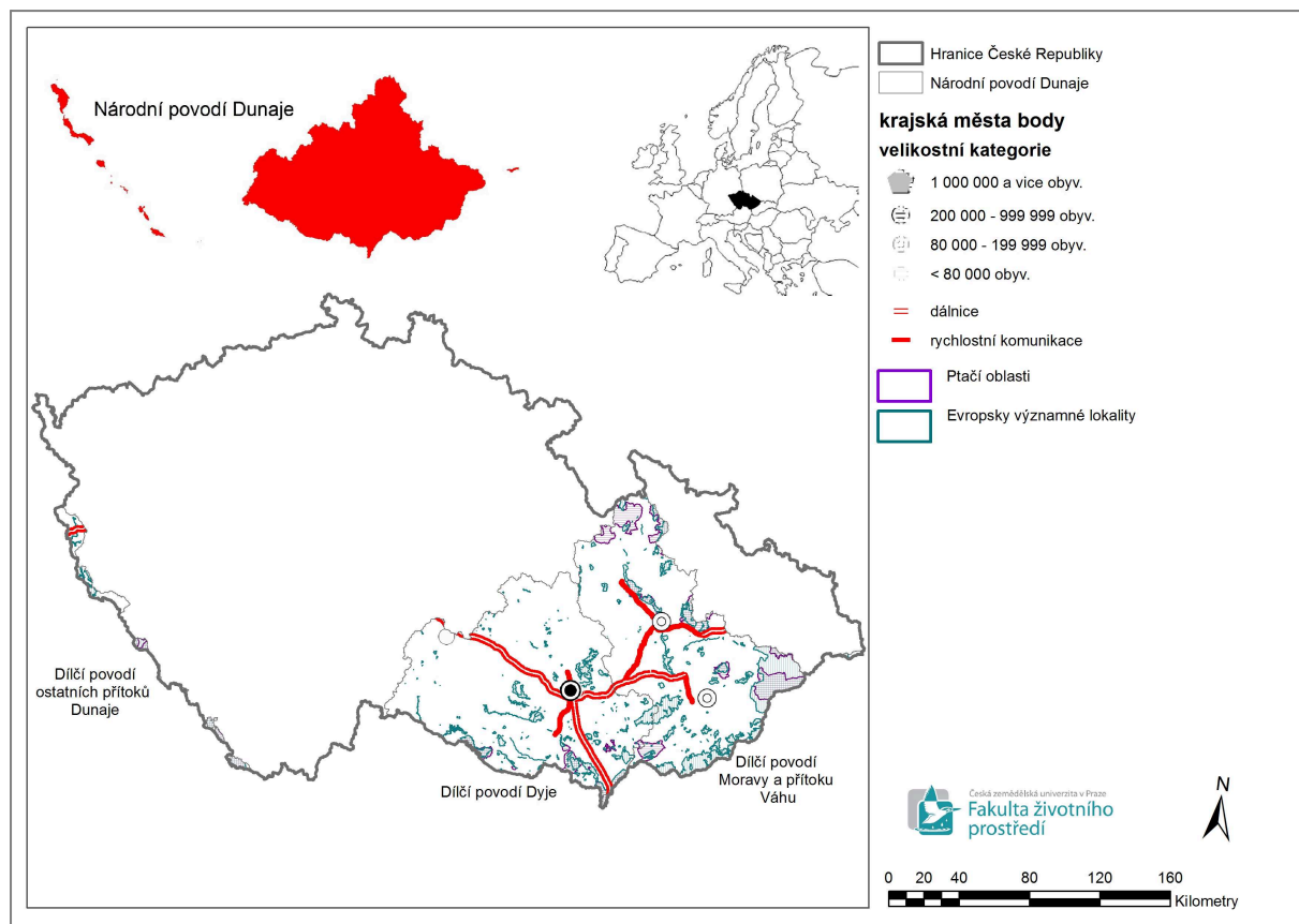
Obrázek č. 20 Území Nature 2000, evropsky významné lokality a ptačí oblasti v roce 2013 v rámci území Plánu pro zvládnání povodňových rizik v povodí Dunaje
