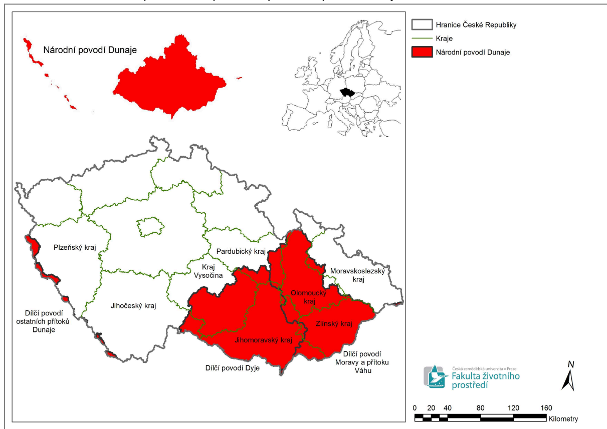
Obrázek č. 2 Území Plánu pro zvládnání povodňových rizik v povodí Dunaje
