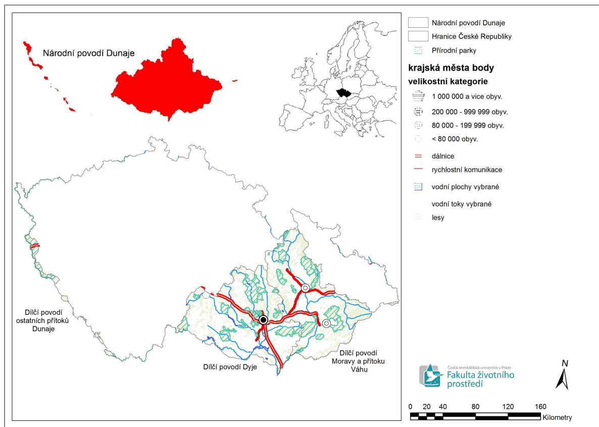
Obrázek č. 22 Přírodní parky v rámci území Plánu pro zvládnání povodňových rizik v povodí Dunaje
