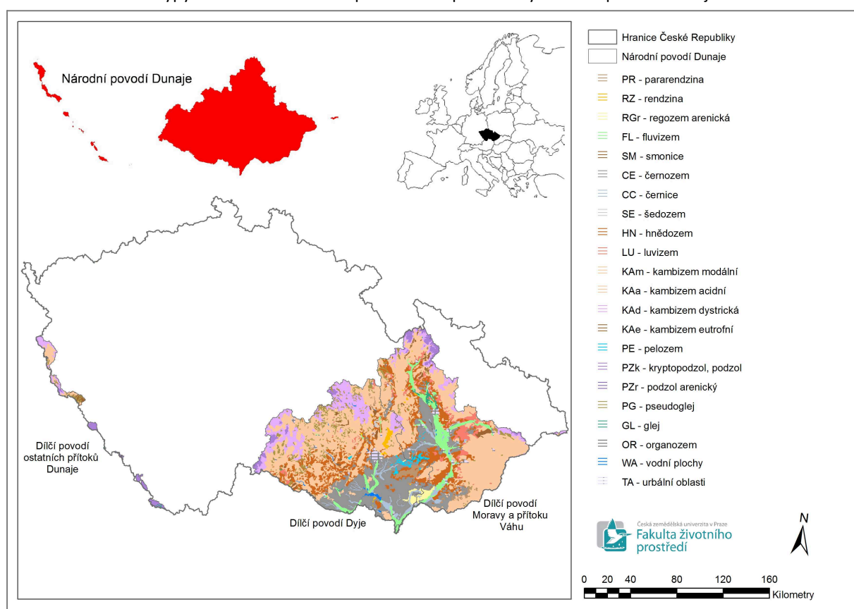
Obrázek č. 17 Půdní typy v rámci území Plánu pro zvládnání povodňových rizik v povodí Dunaje
