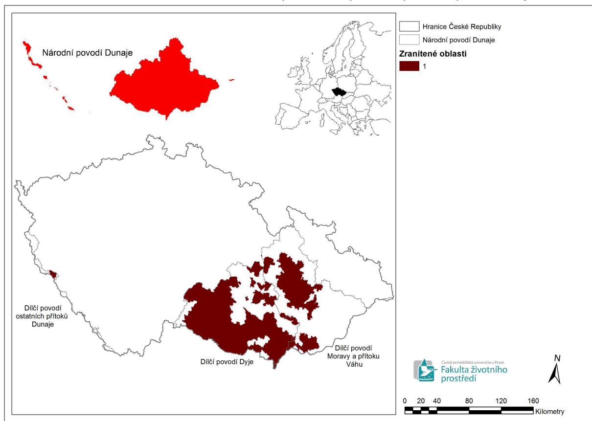
Obrázek č. 12 Zranitelné oblasti v rámci území Plánu pro zvládnutí povodňových rizik v povodí Dunaje
