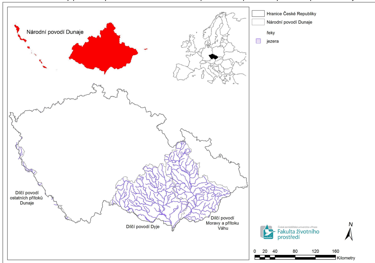
Obrázek č. 10 Útvary povrchových vod v rámci území Plánu pro zvládnání povodňových rizik v povodí Dunaje
