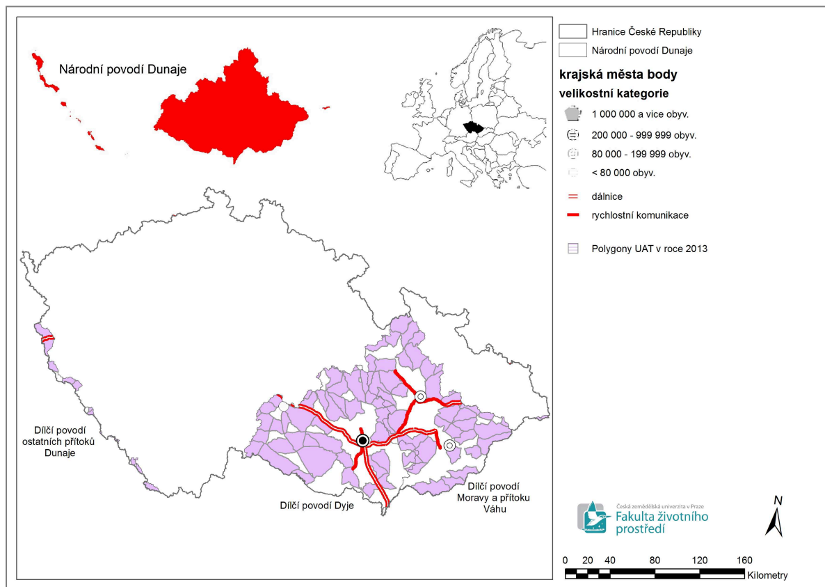
Obrázek č. 23 Fragmentace krajiny (UAT) v roce 2013 v rámci území Plánu pro zvládnání povodňových rizik v povodí Dunaje
