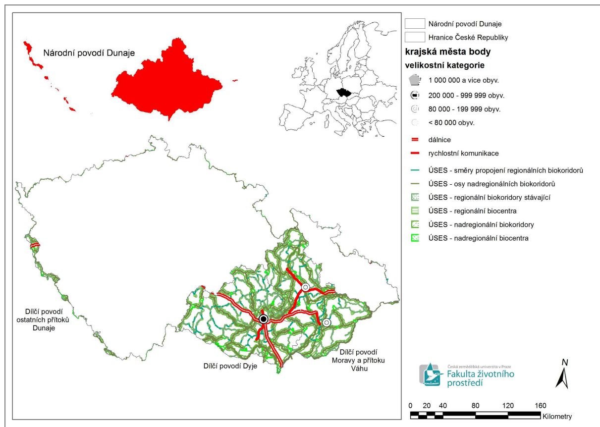
Obrázek č. 25 Územní systém ekologické stability v rámci území Plánu pro zvládnání povodňových rizik v povodí Dunaje
