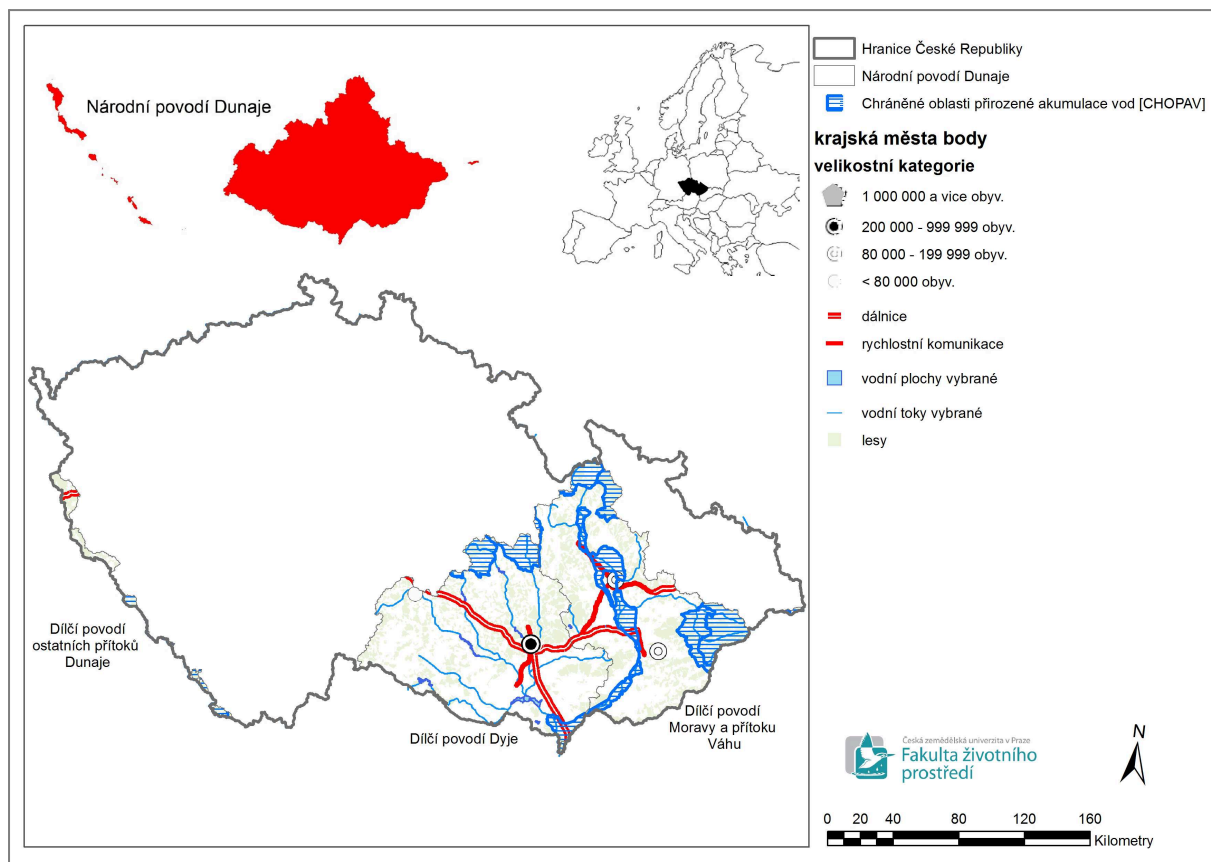
Obrázek č. 13 Chráněné oblasti přirozené akumulace vod v rámci území Plánu pro zvládnutí povodňových rizik v povodí Dunaje
