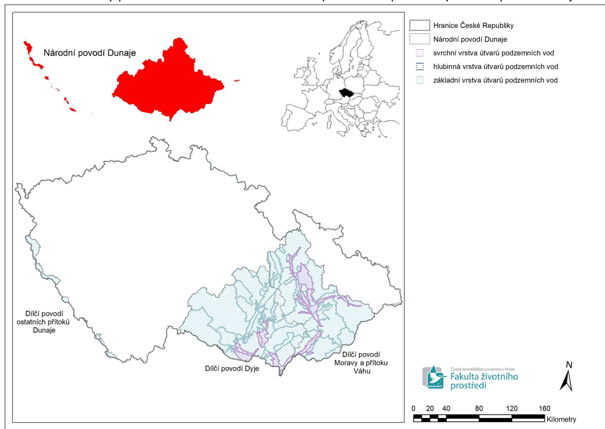
Obrázek č. 11 Útvary podzemních vod v rámci území Plánu pro zvládnání povodňových rizik v povodí Dunaje
