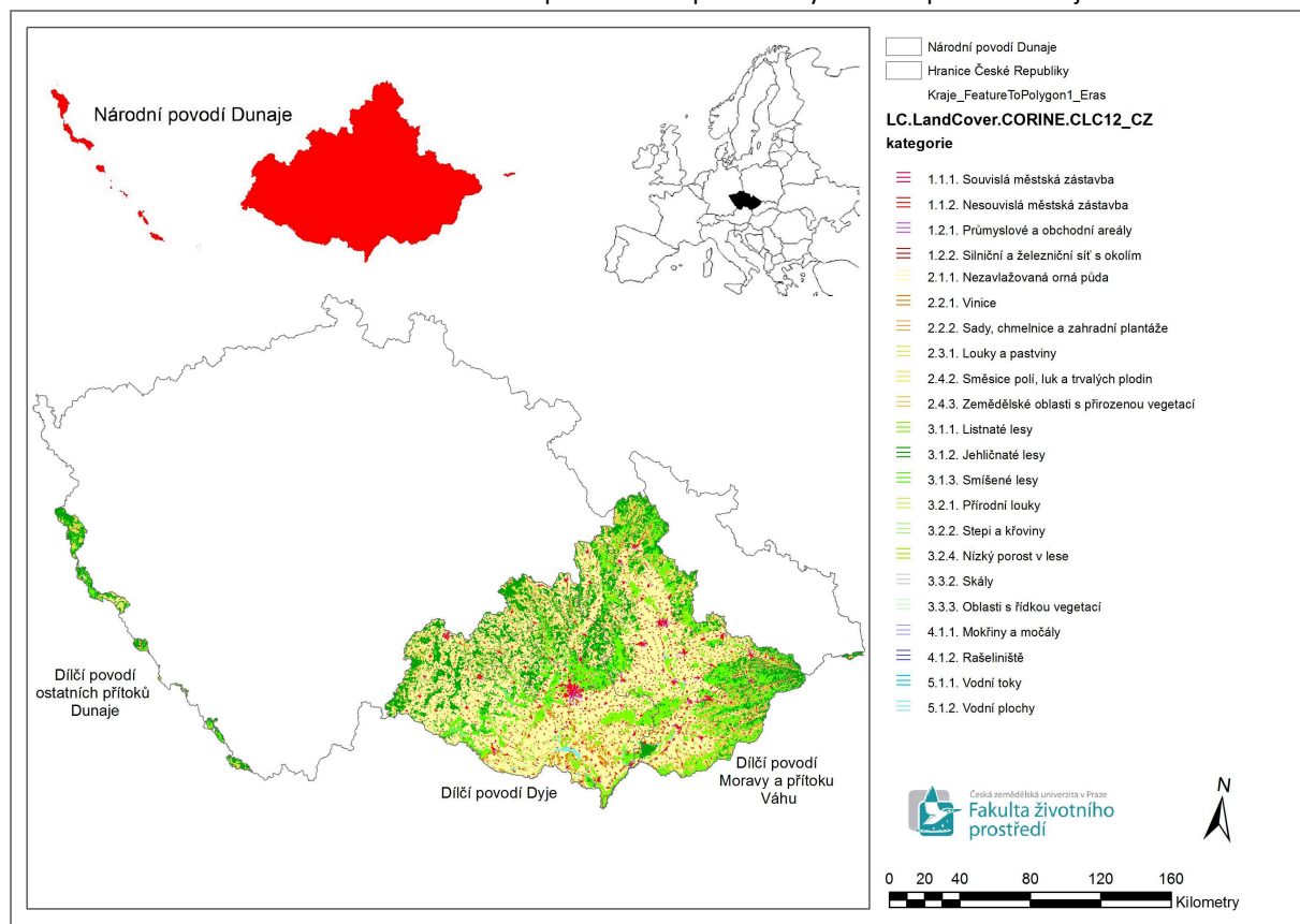
Obrázek č. 18 Land cover v rámci území Plánu pro zvládnání povodňových rizik v povodí Dunaje
