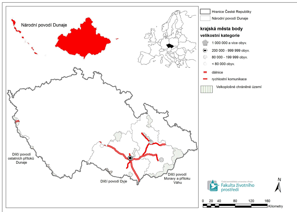
Obrázek č. 19 Velkoplošná chráněná území v rámci území Plánu pro zvládnání povodňových rizik v povodí Dunaje
