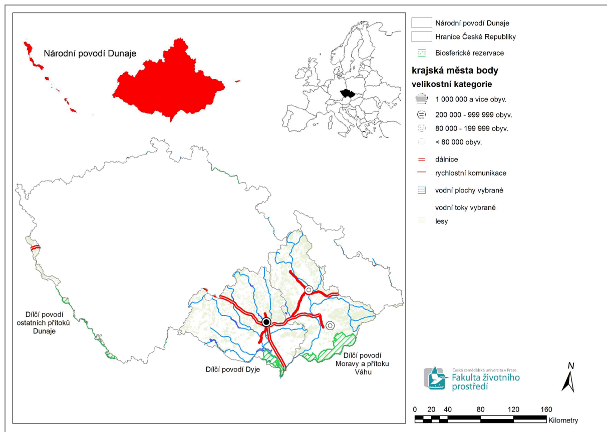
Obrázek č. 21 Biosférické rezervace v rámci území Plánu pro zvládnutí povodňových rizik v povodí Dunaje
